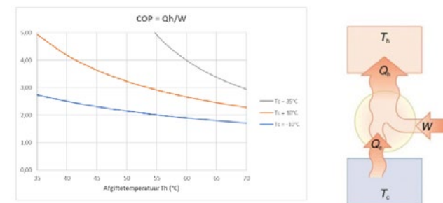
Indicatieve COP voor warmtepompen in verschillende temperatuurregimes.
