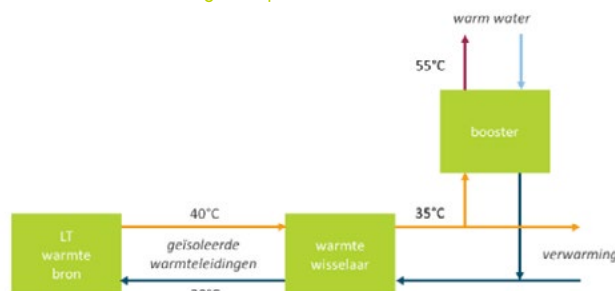
Lage temperatuur-warmtenet
